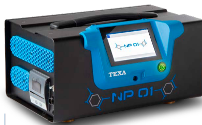
NP 01 je prvo orodje TEXA nove generacije instrumentov, razvito in zasnovano za merjenje koncentracije delcev v emisijah motornih vozil.
